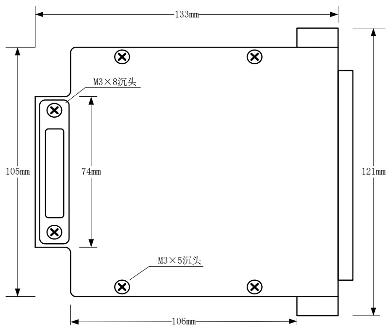
图 3-2-2 TB8091 板卡尺寸图
