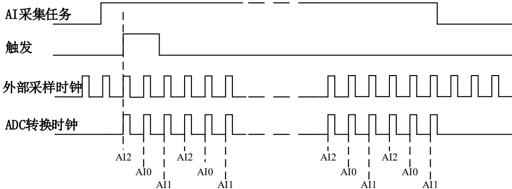
图4-8-5 外时钟连续采样
