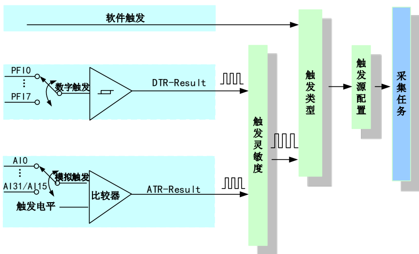
图 8-1-1 触发源选择
