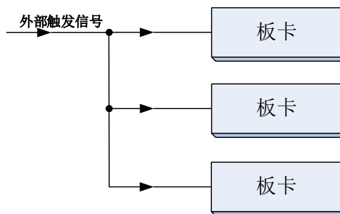
图 4-10-3 外触发同步采集的连接方式
