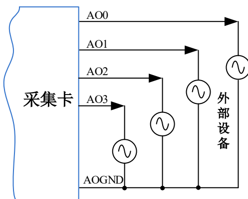
图5-2-1 AO模拟量输出连接
