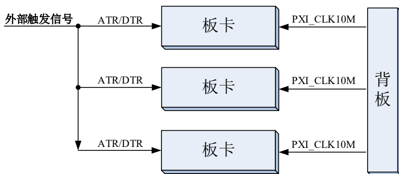
图 4-10-1 主从卡级联
