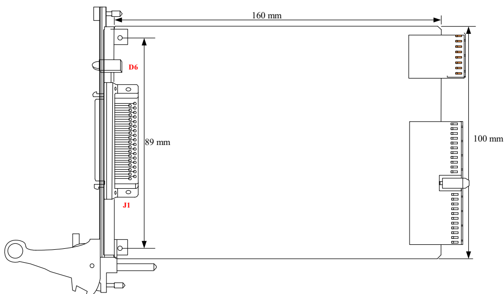
图 3-2-1 外壳尺寸图
