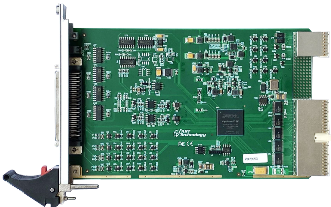
图 3-1-1 PXI5650/1/2/3/4/5/6/7 正面图
